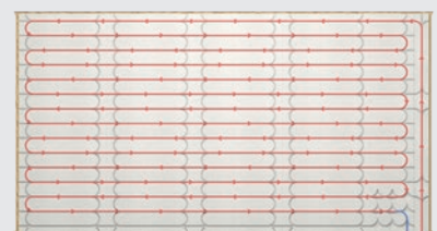
Verlegung der Heizrohre (16 mm)
