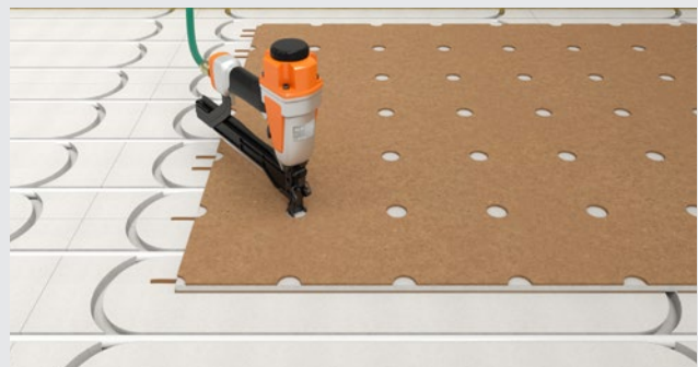
Montage der Abdeckplatte und mechanische Befestigung mittels Schrauben oder Klammern unter Verwendung der Schablone.
