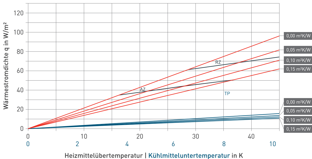
Kennliniendiagramm Heizen und Kühlen fermacell® Therm 25™-125, MKV 16×2, VA = 250 mm
