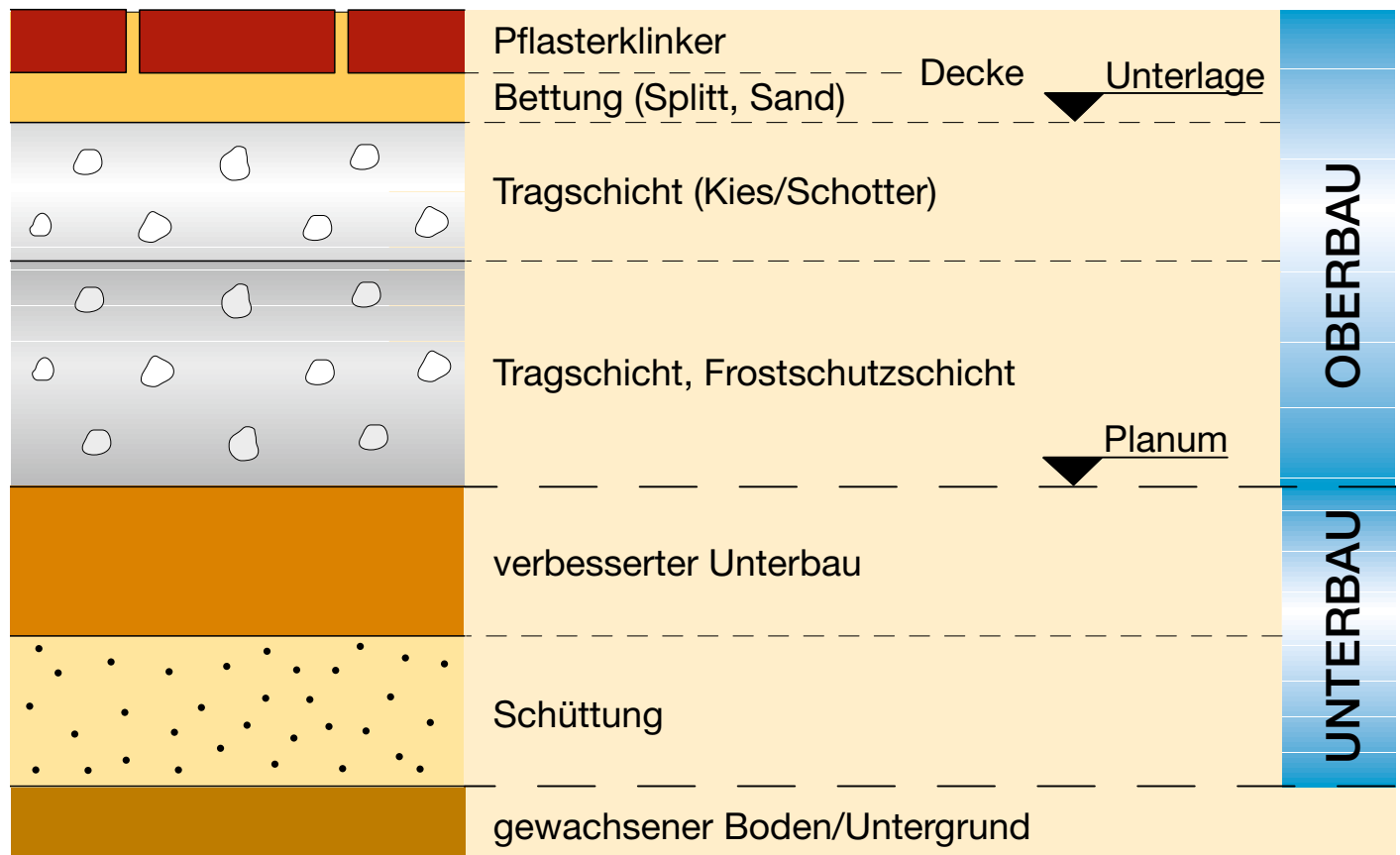
Aufbaubeispiel einer Verkehrsflächenbefestigung mit Pflasterklinkern
